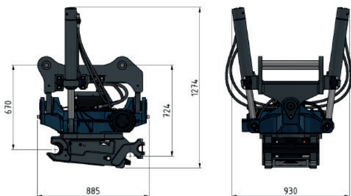
Dimensioner för ST28 med S70 Hardlock
