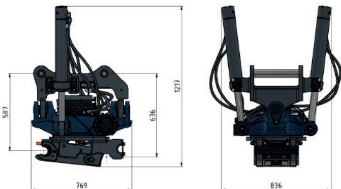
Dimensioner för ST18 med S60 Hardlock
