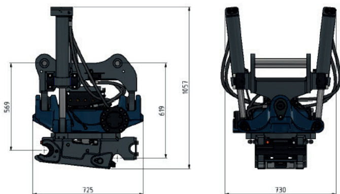
Dimensioner för ST15 med S60 Hardlock
