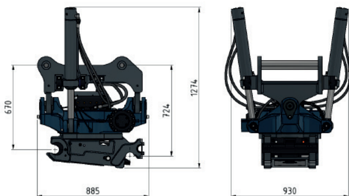
Dimensjoner for ST32 med S70 Hardlock.
