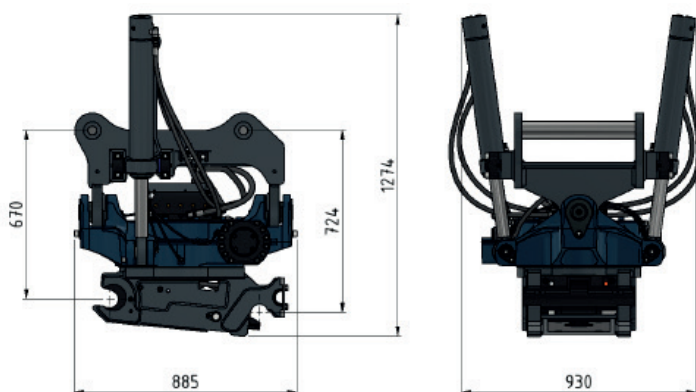
Dimensjoner for ST28 med S70 Hardlock
