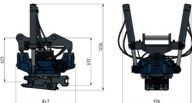
Dimensjoner for ST22 med S60 Hardlock
