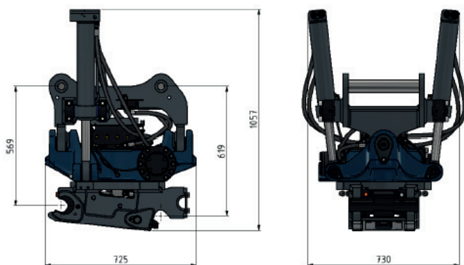
Dimensioner for ST15 med S60 Hardlock
