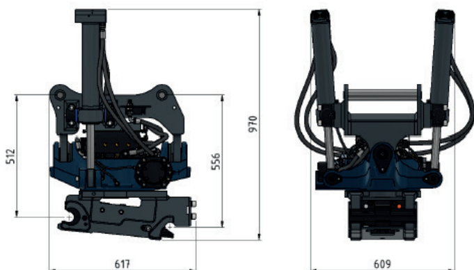
Dimensjoner for ST10 med S45 Hardlock
