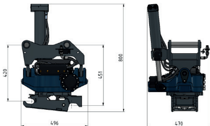
Dimensjoner för ST6 med S40 Safelock
